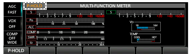
Visualizado cuando la función Peak Hold está activada.
