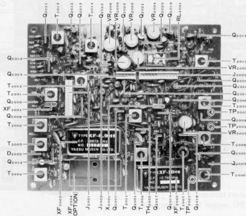
IF UNIT
