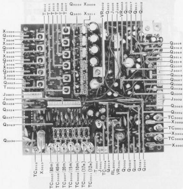
AF UNIT
